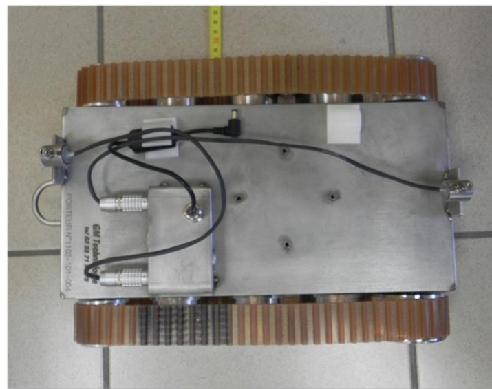
Porteur d'acheminement scan 3D HADE La Hague
