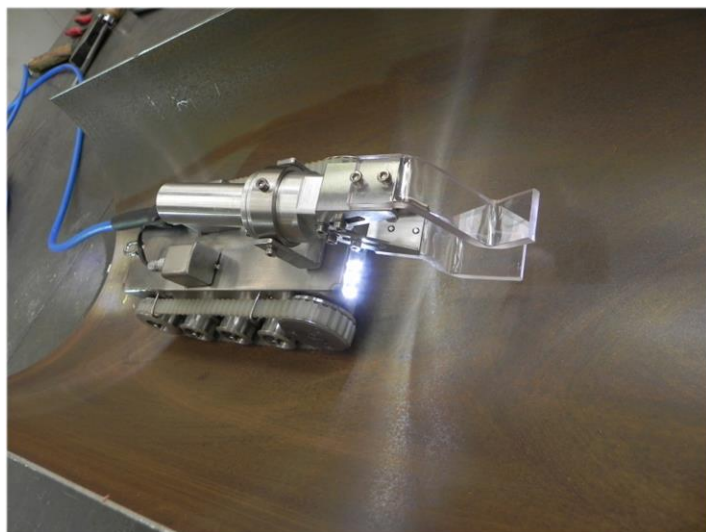
Porteur de récupération de débris dans une tuyauterie diamètre 400mm EDF Flamanville
