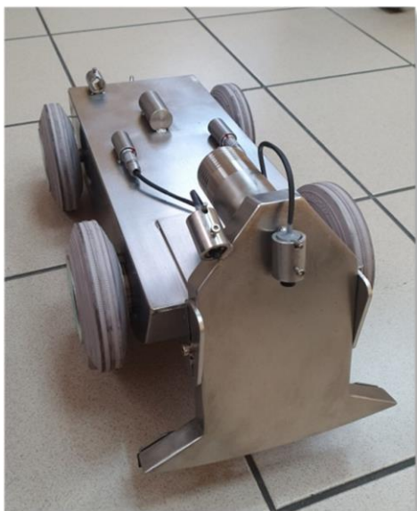
Porteur d'assainissement cuve EDF Chinon
