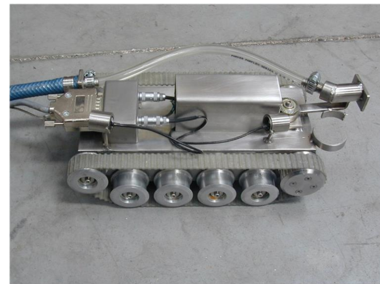
Porteur de nettoyage aspiration
