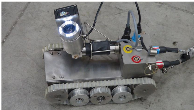
Porteur de visualisation, mesure laser, prise d'échantillons HAO La Hague
