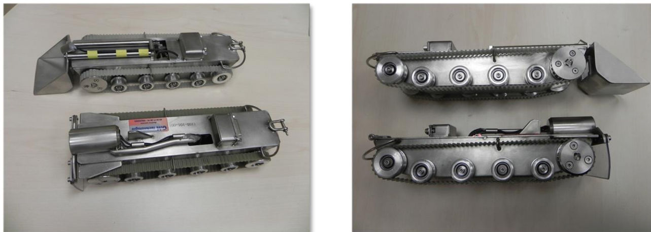
Porteurs d'investigation vidéo et de prélèvement solide
