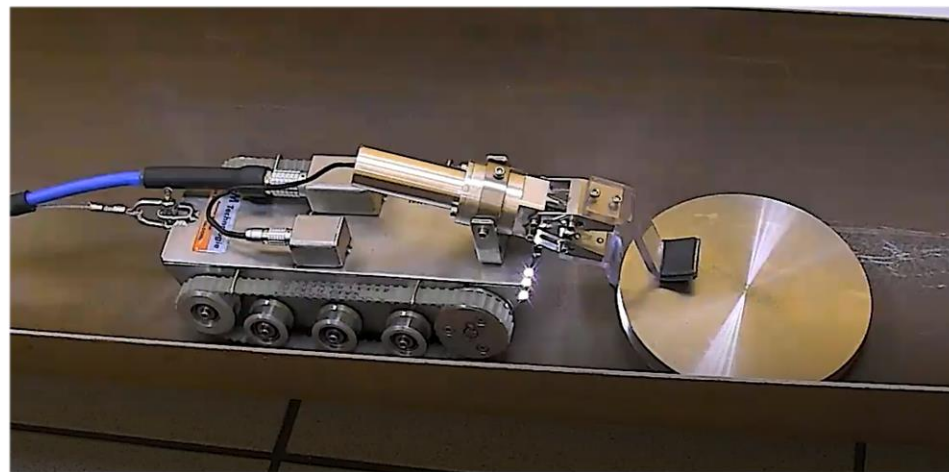
Porteur de récupération de débris dans une tuyauterie diamètre 400mm EDF Flamanville
